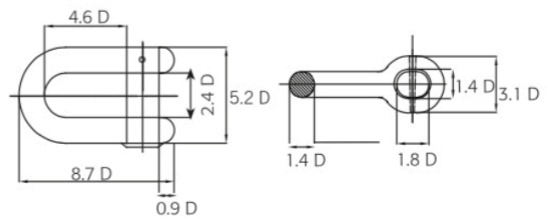
MANILHA DE ANCORA TIPO "D"
